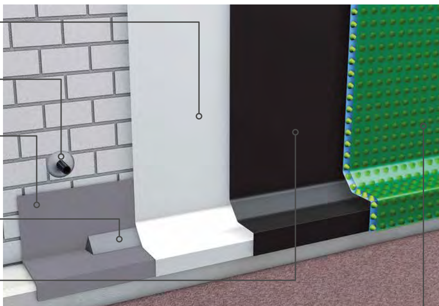
Systeemvoorbeeld: Afdichting volgens DIN EN 18 533
